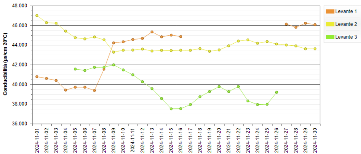
Figura 12 - Andamento medio giornaliero della Conducibilità nella Laguna di Levante.
