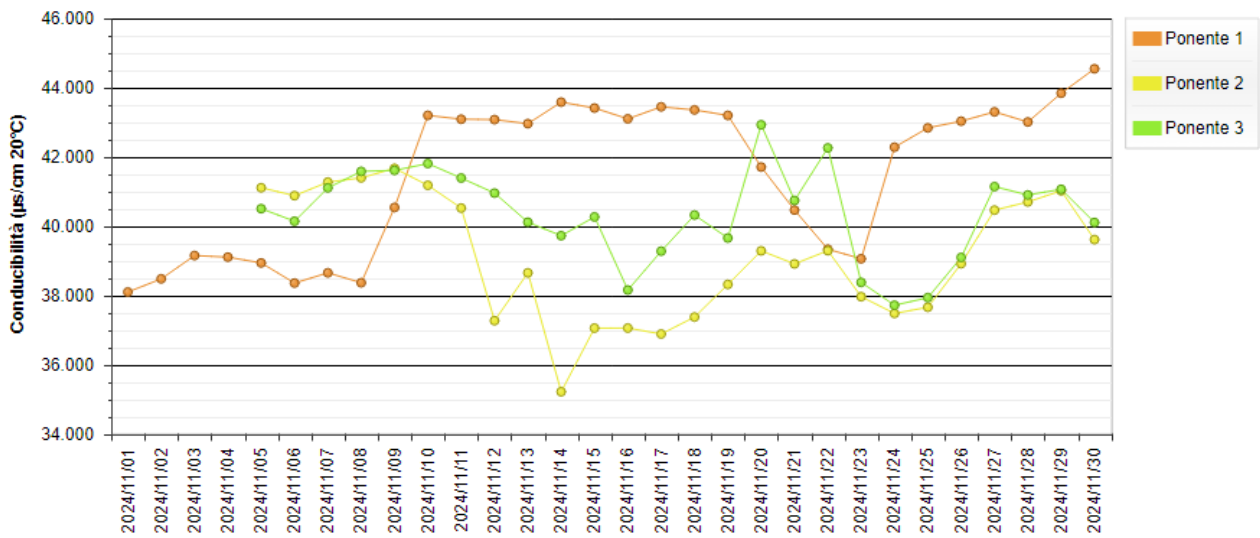
Figura 11 - Andamento medio giornaliero della Conducibilità nella Laguna di Ponente.
