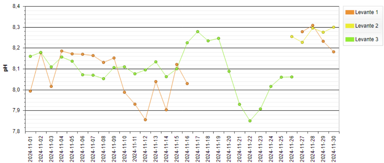
Figura 10 – Andamento medio giornaliero del pH nella Laguna di Levante.
