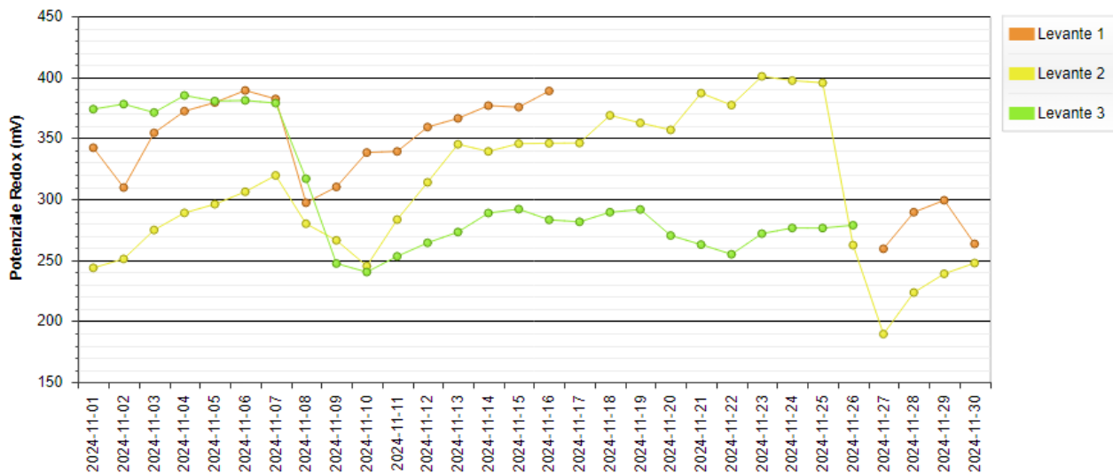
Figura 14 - Andamento medio giornaliero del Potenziale Redox nella Laguna di Levante.
