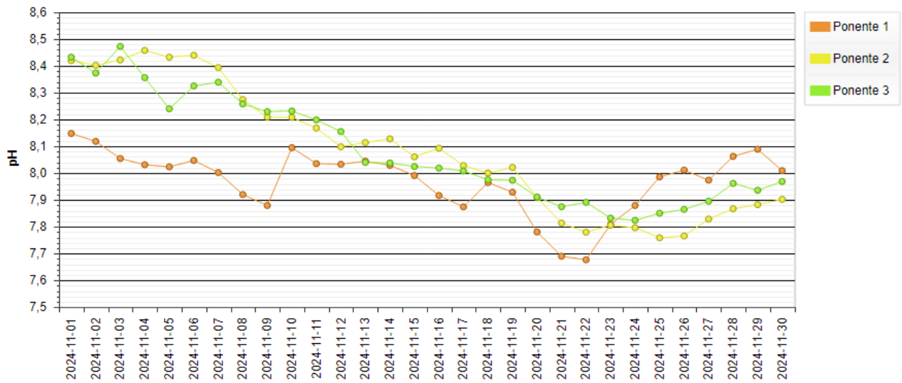
Figura 9 – Andamento medio giornaliero del pH nella Laguna di Ponente.
