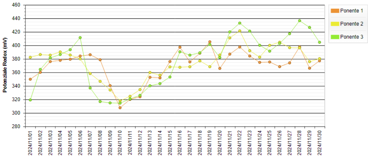
Figura 13 - Andamento medio giornaliero del Potenziale Redox nella Laguna di Ponente.
