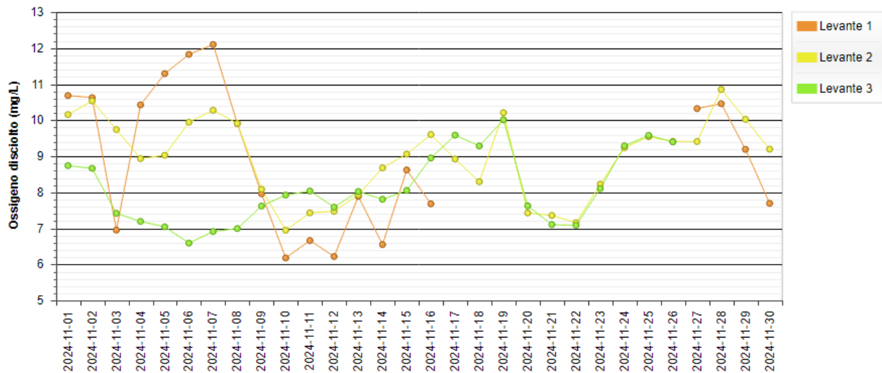
Figura 18 - Andamento medio giornaliero dell'Ossigeno disciolto nella Laguna di Levante.
