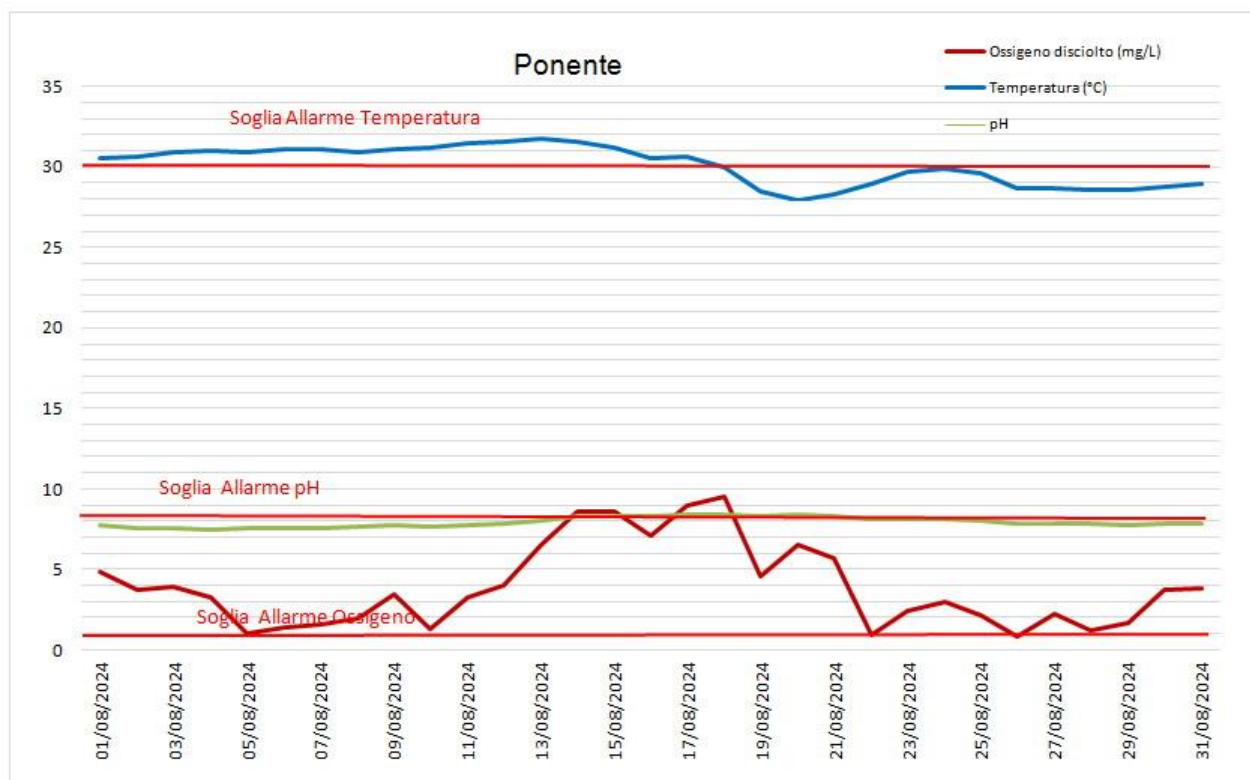
Figura 13 - Andamento medio giornaliero e Soglie di Allarme per i parametri Temperatura, pH ed Ossigeno disciolto registrati dalla sonda multiparametrica Ponente.
