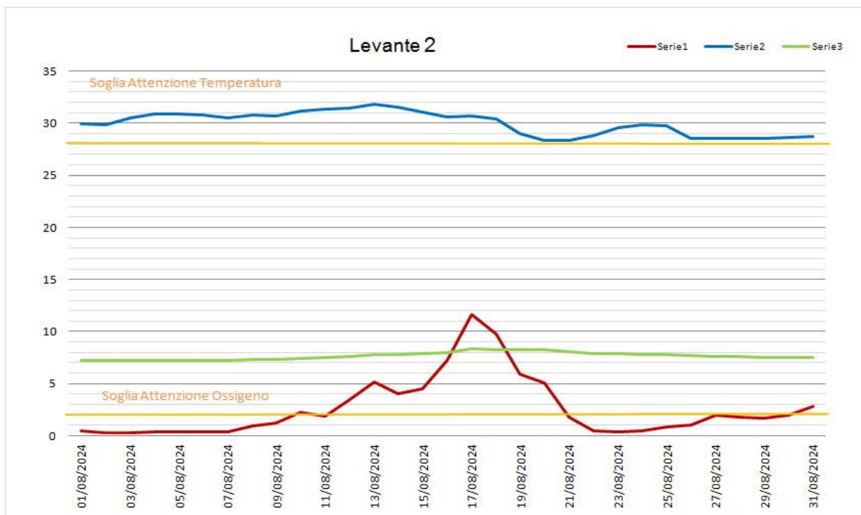
Figura 10 - Andamento medio giornaliero e Soglie di Attenzione per i parametri Temperatura, pH, Ossigeno disciolto registrati dalla sonda multiparametrica Levante 2. Il pH non presenta Soglie di Attenzione (ma solo di Allarme).
